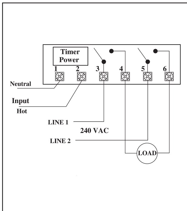
FIG. #5 ET104C DPST
