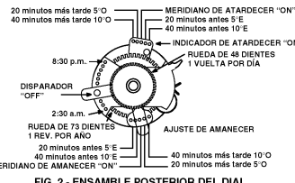
FIG. 2 - ENSAMBLE POSTERIOR DEL DIAL
